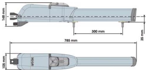
413规格尺寸
